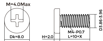
벽걸이 나사 사양: M4*(10+X)mm (X=벽걸이 브래킷 두께)
