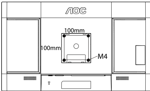
벽걸이 나사 사양: M4*(10+X)mm (X=벽걸이 브래킷 두께)
