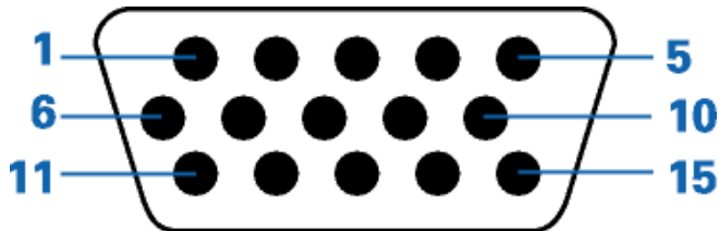
15-poliges Farbdisplay-Signalkabel
