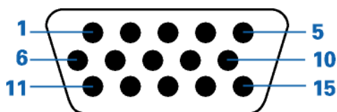
15-stykowy przewód sygnałowy kolorowego wyświetlacza
