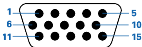
15-изводен сигнален кабел за цветен монитор
