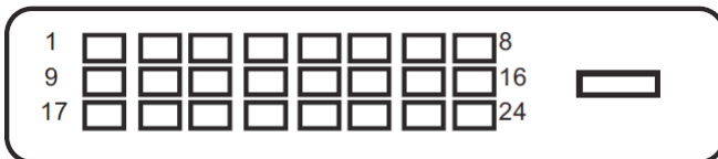
24-stykowy przewód sygnałowy kolorowego wyświetlacza
