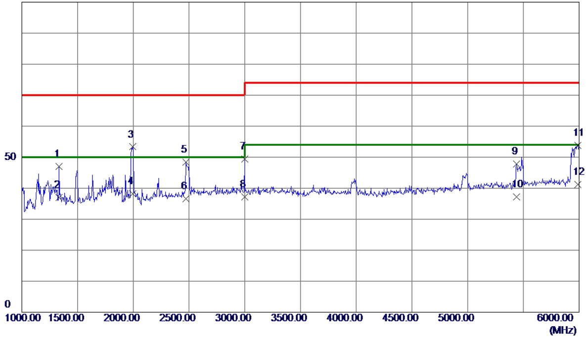
100 dBuV/m
