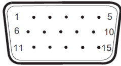
15-nastainen värinäyttösignaalikaapeli
