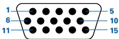
15-изводен сигналел кабел за цветен монитор
